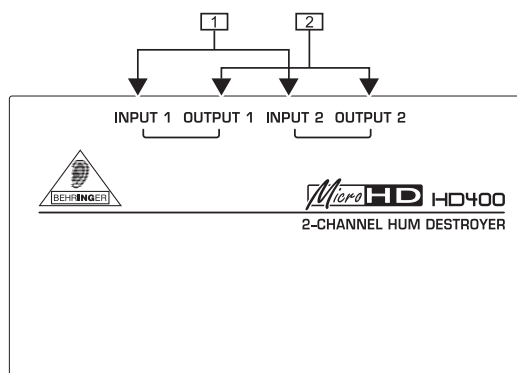
Collegamenti del HD400
