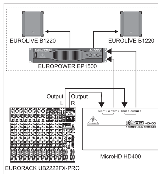
Cablaggio del HD400
