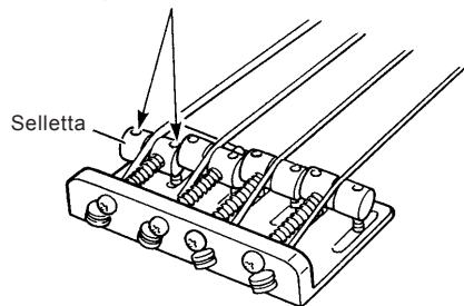
Regolazione altezza
